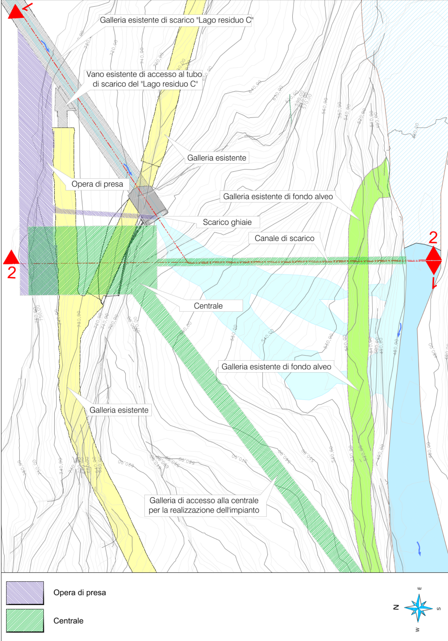
PLANIMETRIA
